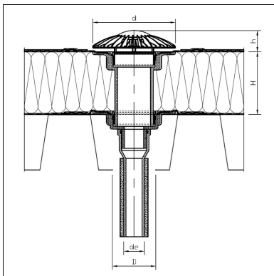
Warmdach, frei bewittert, Leichtbau, SDA-Speed, PE-HD Steckmuffe
