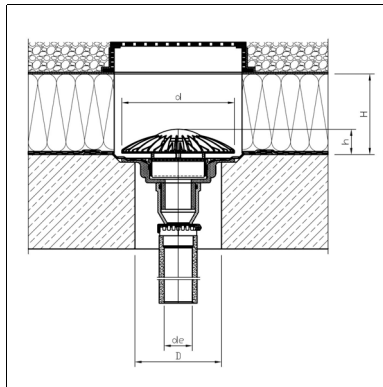
Umkehdach, Kies, Massivdach, SDA-Speed, PE-HD Steckmuffe auf PK-NG Rohr
