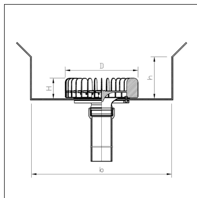
Rinne, VA-Dachablauf mit Gegenflansch, PE-HD Anschlussstutzen
