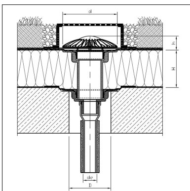
Warmdach, begrünt, Massivdach, SDA-Speed, PE-HD Steckmuffe
