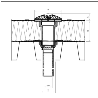
Warmdach, frei bewittert, Leichtbau, SDA-Speed, PK-NG Rohr
