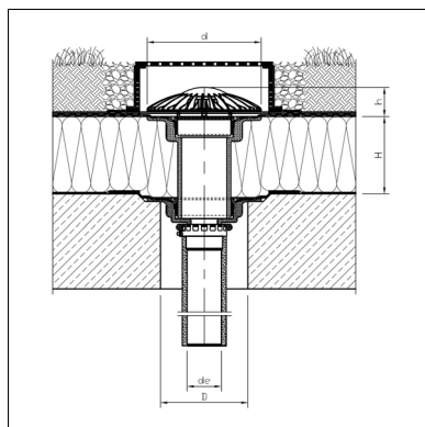
Warmdach, begrünt, Massivdach, SDA-Speed, PK-NG Rohr
