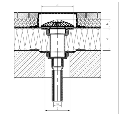
Warmdach, begehbar (Terrasse), Massivdach, SDA-Speed, PE-HD Steckmuffe
