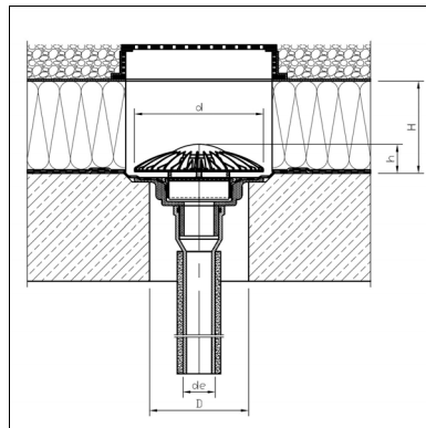
Umkehrdach, Kies, Massivdach, SDA-Speed, PE-HD Steckmuffe
