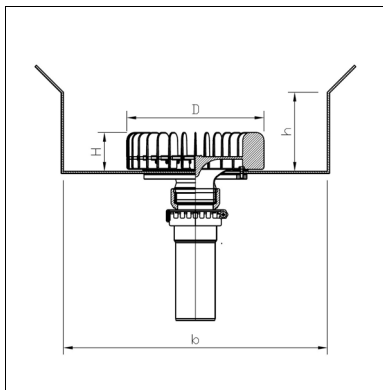
Rinne, VA-Dachablauf mit Gegenflansch, PE-HD Anschlussstutzen auf PK-NG Rohr
